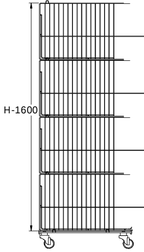
AKSİYON SEPET DÜZ STACKING WIRE BASKET
