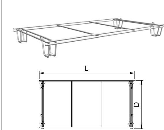
AKSİYON SEPET ALTLIĞI TEL STACKING WIRE BASKET BASE WIRE
