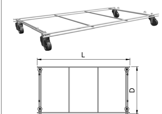
AKSİYON SEPET ALTLIĞI TEL TEKERLEKLİ STACKING WIRE BASKET BASE WIRE MOBILE
