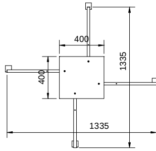
GOVDE / MAIN FRAME
