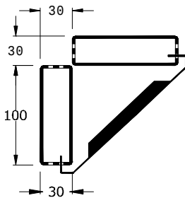
DIŞ KÖŞE YERLEŞİM ÖLÇÜLERİ EXTERNAL CORNER SIZES
