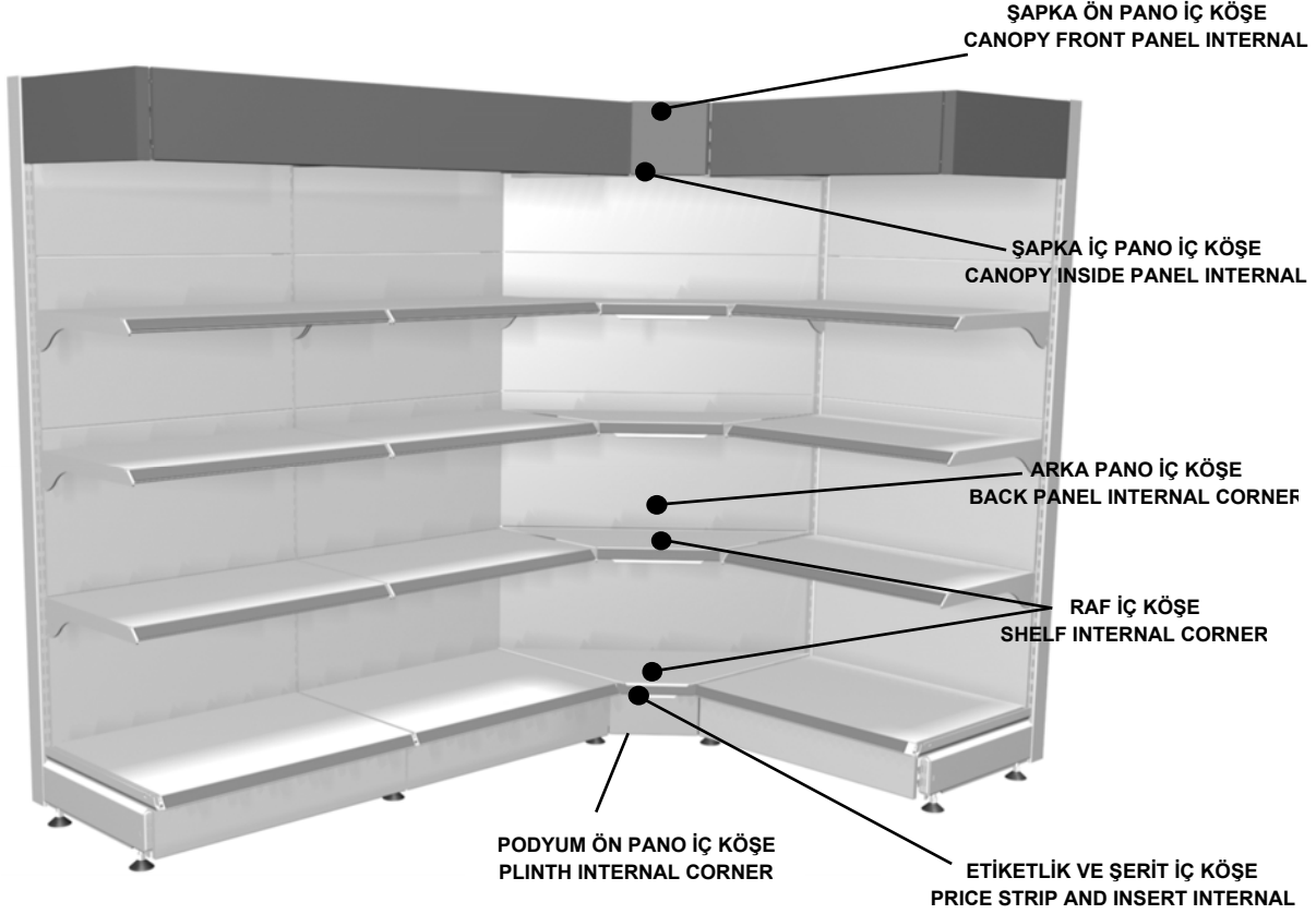
İÇ KÖŞE REYON INTERNAL CORNER UNIT
