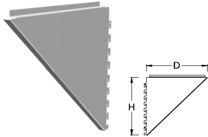
ŞAPKA YAN PANO SAĞ MEY MEY CANOPY SIDE PANEL RIGHT
