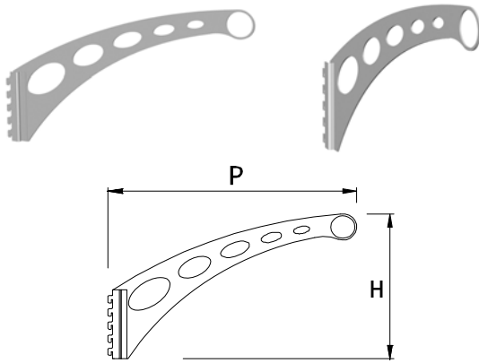
AYDINLATMA KONSOLU TİP 1 ILLUMINATION BRACKET TYPE 1
