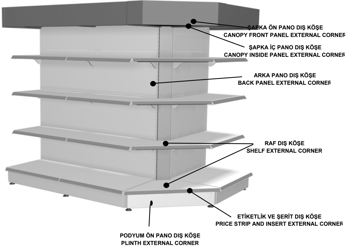
DIŞ KÖŞE REYON EXTERNAL CORNER UNIT
