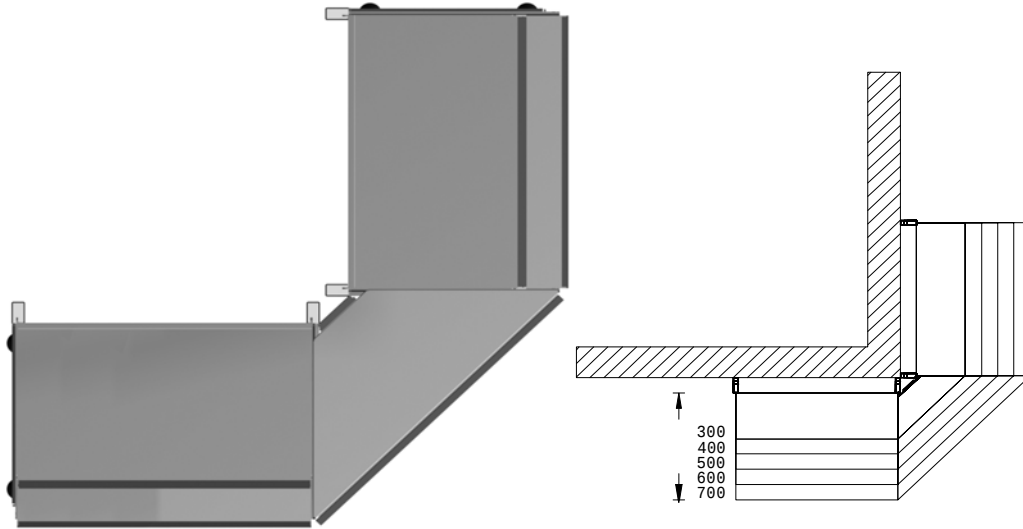
DIŞ KÖŞE REYON EXTERNAL CORNER UNIT
