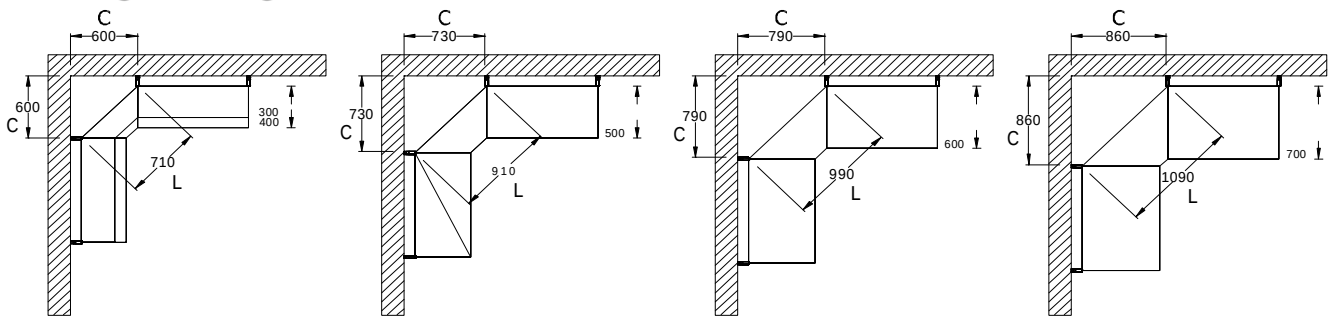
İÇ KÖŞE YERLEŞİM ÖLÇÜLERİ INTERNAL CORNER SIZES
