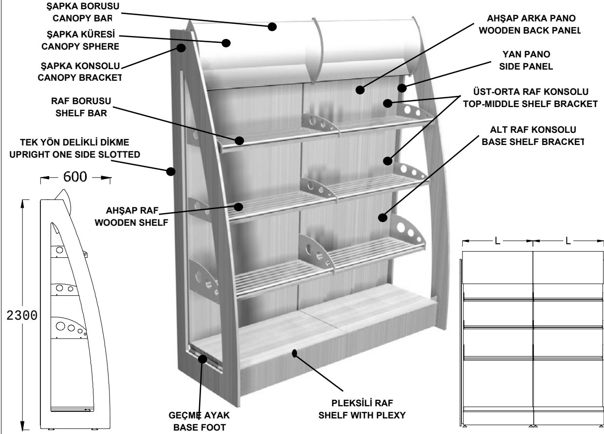
UM5 UNLU MAMUL REYONU UM5 BAKERY UNIT
