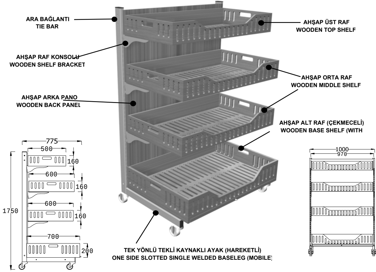
UM7 UNLU MAMUL REYONU UM7 BAKERY UNIT
